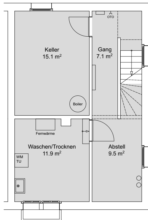
Untergeschoss
