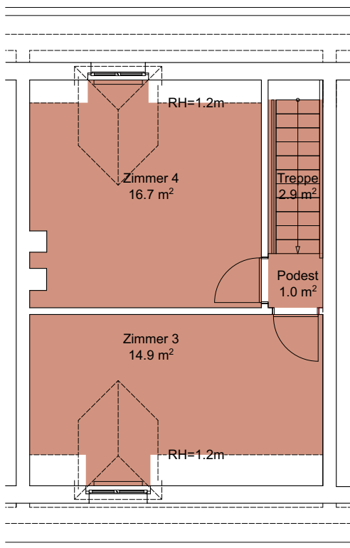
Grundriss DG
