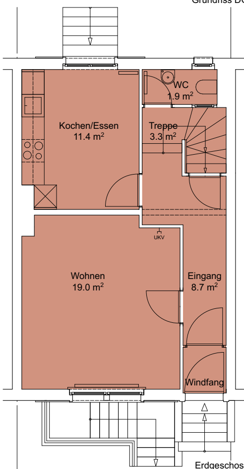
Erdgeschoss
