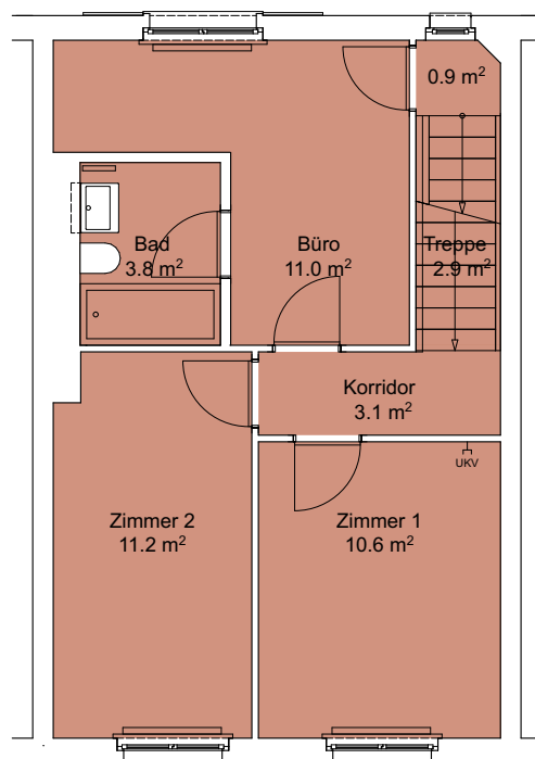
Obergeschoss
