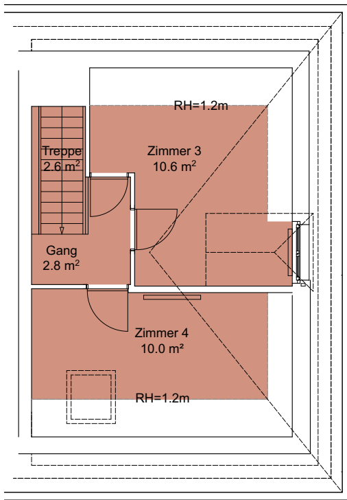
Dachgeschoss
