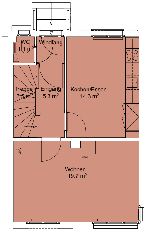
Erdgeschoss
